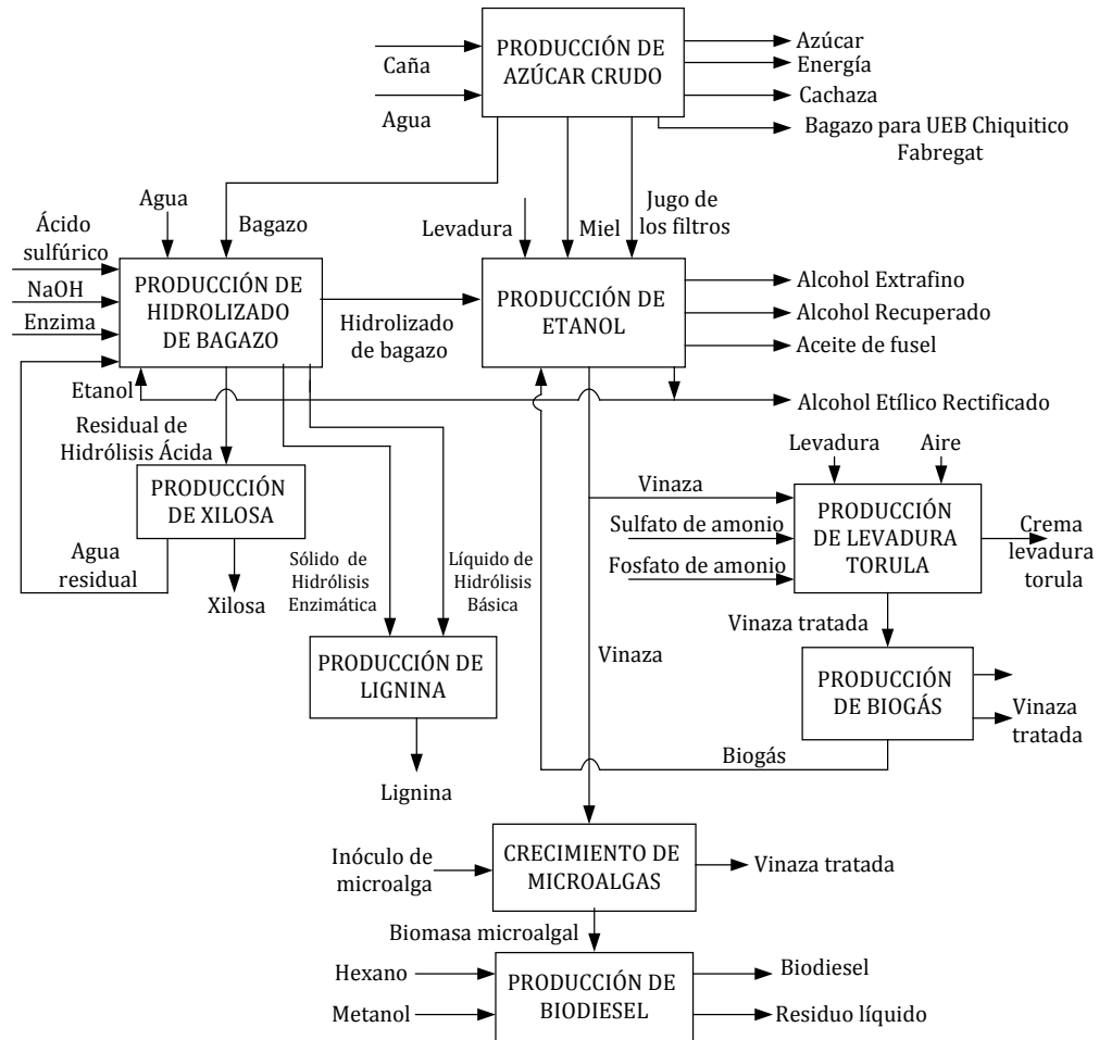
Figura 4. Esquema de integración de la lignina en la biorrefinería
