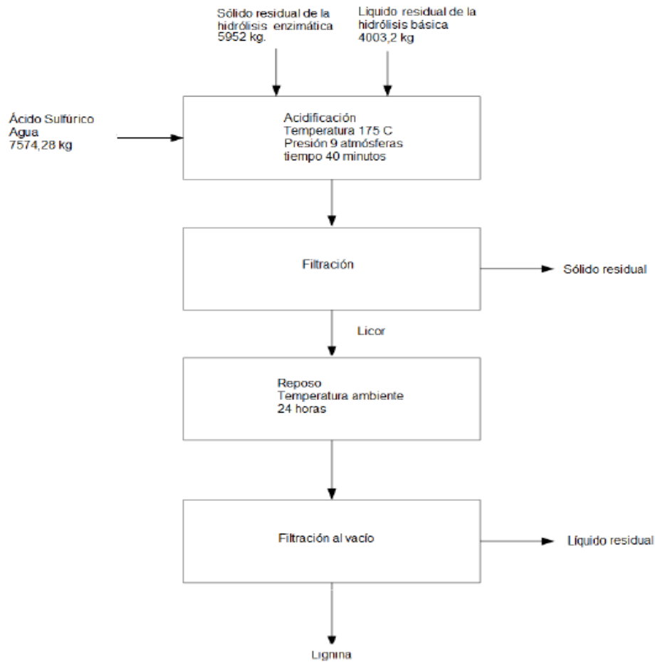
Figura 3. Esquema del proceso (Guirola y Villanueva, 2020)
