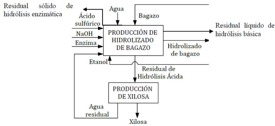
Figura 2. Proceso propuesto para hidrólisis del bagazo (de Armas, 2019)
