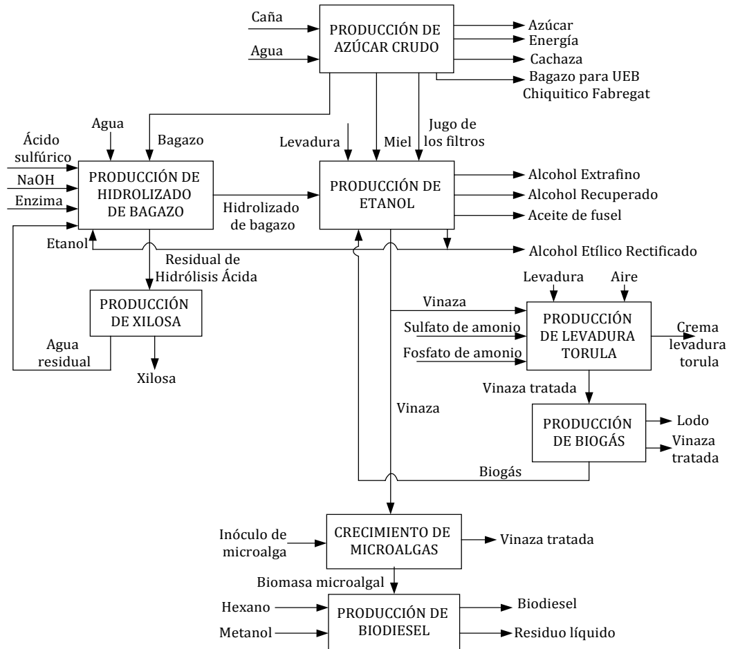
Figura 1. Esquema de biorrefinería integrada de tercera generación (de Armas, 2019)
