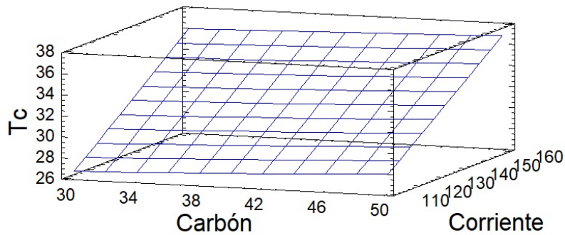
Figura 1. Tasa de consumo (g/min) en función del contenido de carbón de marabú (%) en el revestimiento periférico y de la corriente de soldadura (A)
