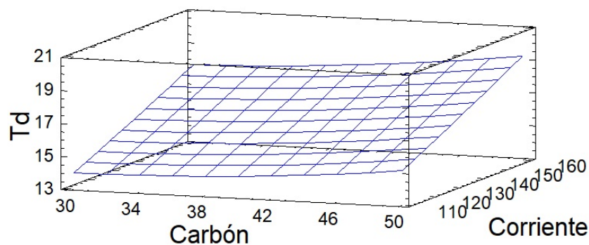
Figura 2. Tasa de deposición (g/min) en función del contenido de carbón de marabú (%) en el revestimiento periférico y de la corriente de soldadura (A)
