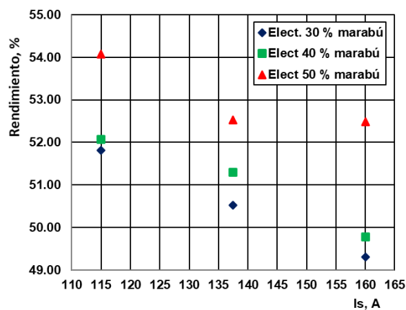
Figura 3. Rendimiento (g/min) en función del contenido de carbón de marabú (%) en el revestimiento periférico y de la corriente de soldadura (A) (a) Gráfico de superficie respuesta; (b) Efecto de la corriente para electrodos con diferentes contenidos de marabú
